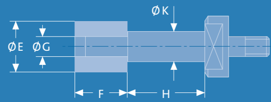
Schleifdorn- und Schleifscheibenabmessungen
